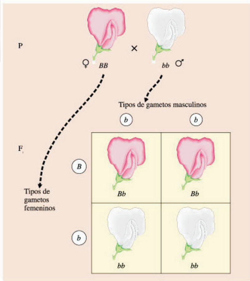
Gráfico 4. Cruzamiento de Prueba
