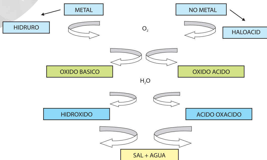
Cuadro de funciones químicas inorgánicas
