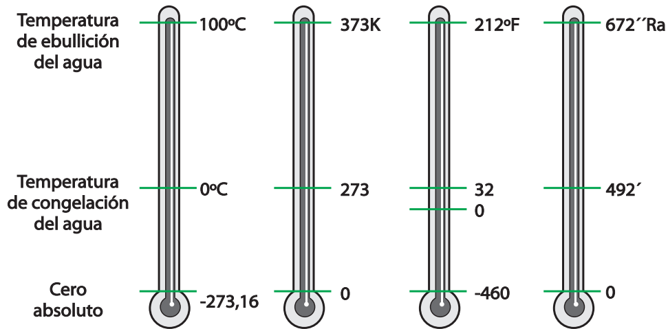
Comparación entre las diferentes escalas de temperatura y los puntos iniciales y finales de la misma
