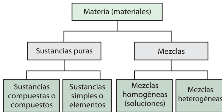
Clasificación de la Materia
