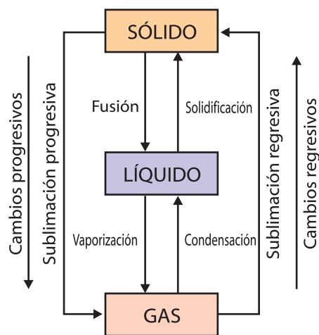
Cambios de estado de la materia
