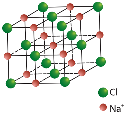
Red cristalina de Cloruro de Sodio
