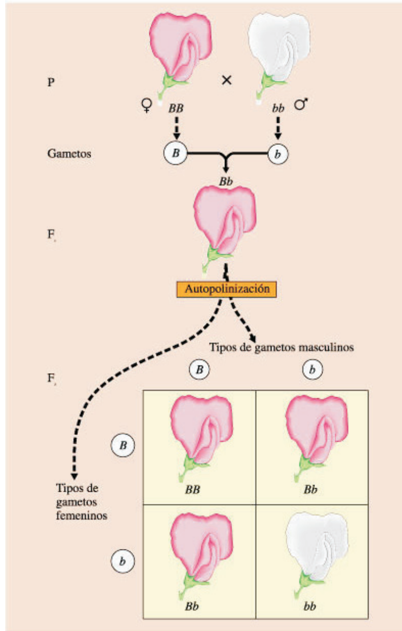
Gráfico 3. Principio de segregación de Mendel
