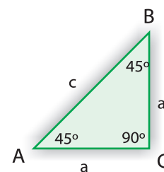
Triángulo isósceles (45 grados)
