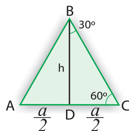
Triángulo equilátero (ángulos 30 y 60 grados)
