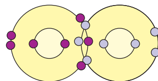
Molécula de nitrógeno Enlace triple (tres pares de electrones compartidos)
