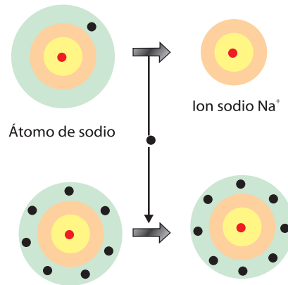
Enlace entre el Ion Sodio y el Ion Cloro
