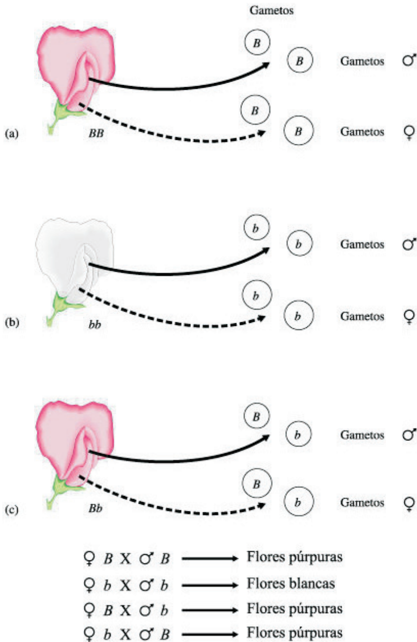
Gráfico 2. Segregación de los Alelos Durante la Formación de los Gametos
