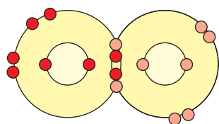
Molécula de oxígeno Enlace doble (dos pares de electrones compartidos)
