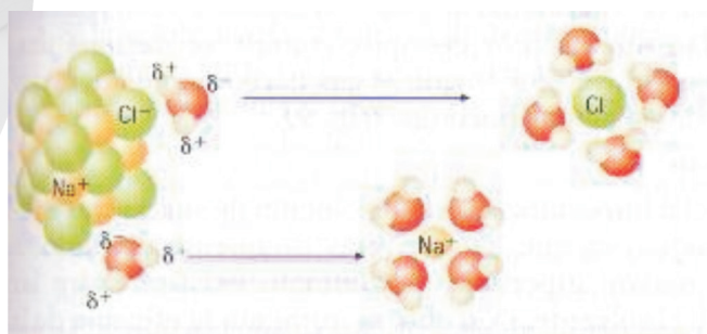
Modelo Ilustrativo del Proceso de Solvatación de Cloruro de Sodio
